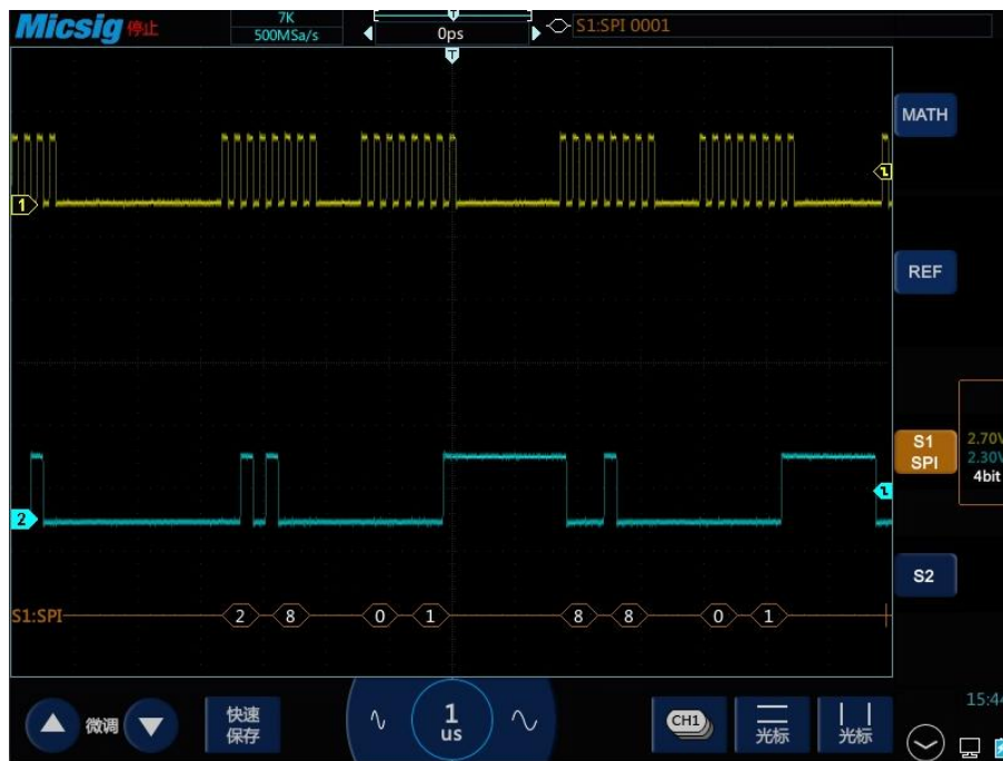
图13-14 SPI 图形界面
