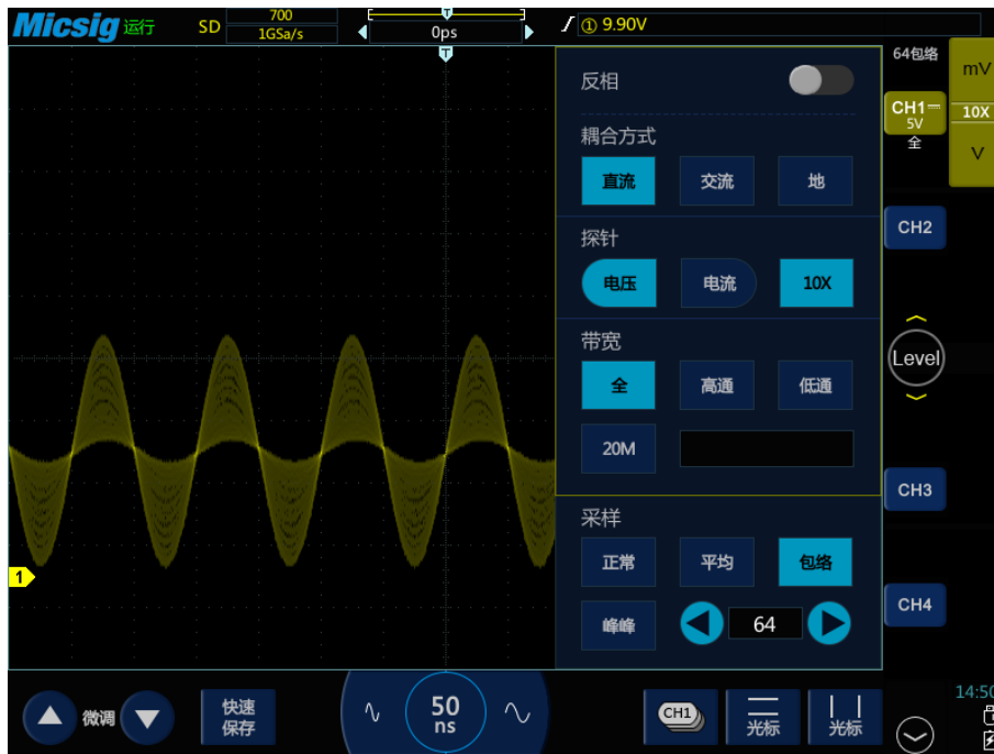
9-8 包络采样模式（64）下的调幅信号
