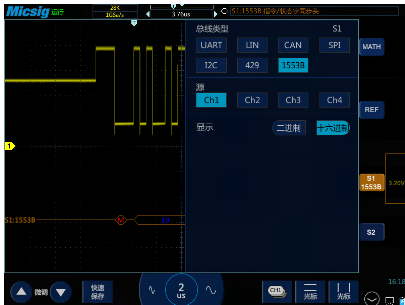
图13-21 1553B 总线配置菜单
