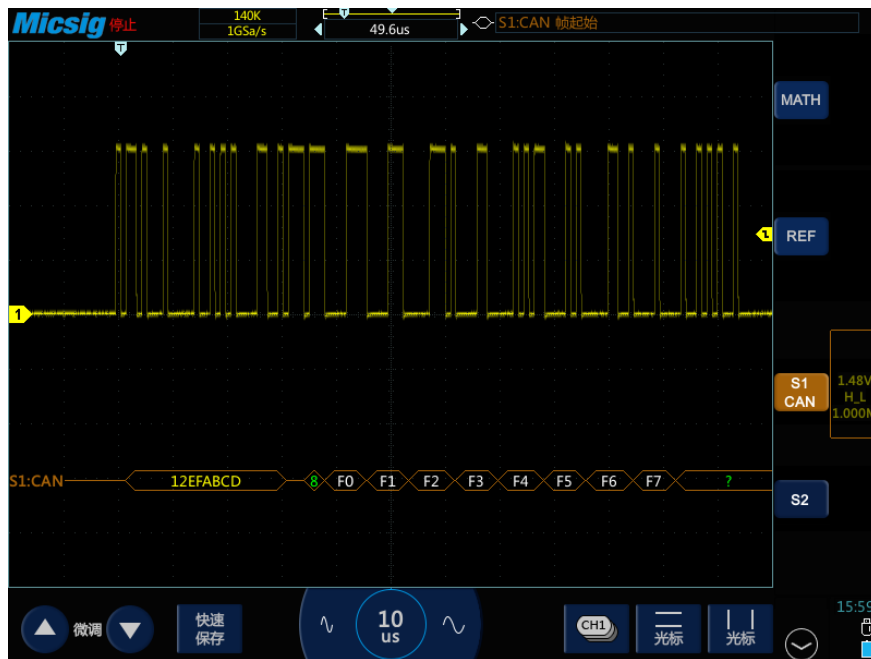
图13-11 CAN 图形界面
