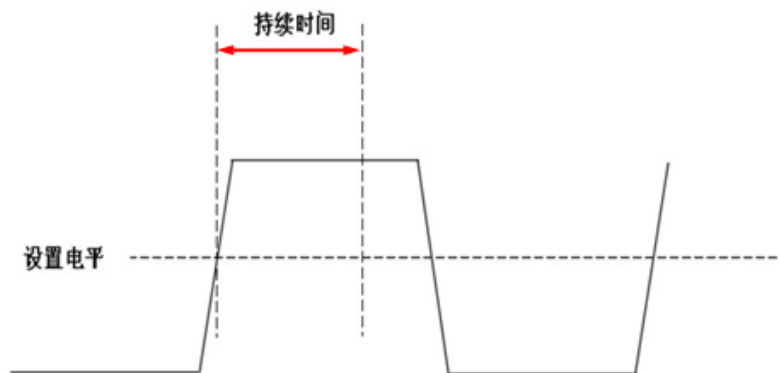
图5-27 超时触发示意图
