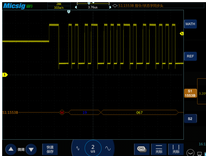
图13-23 1553B 图形界面
