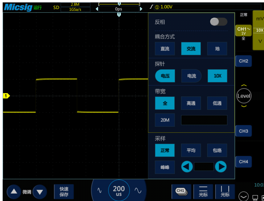
图4-9 AC耦合
