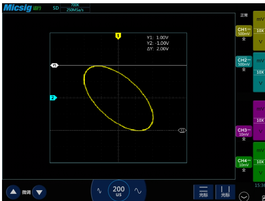
图6-12 XY模式中，光标测量
