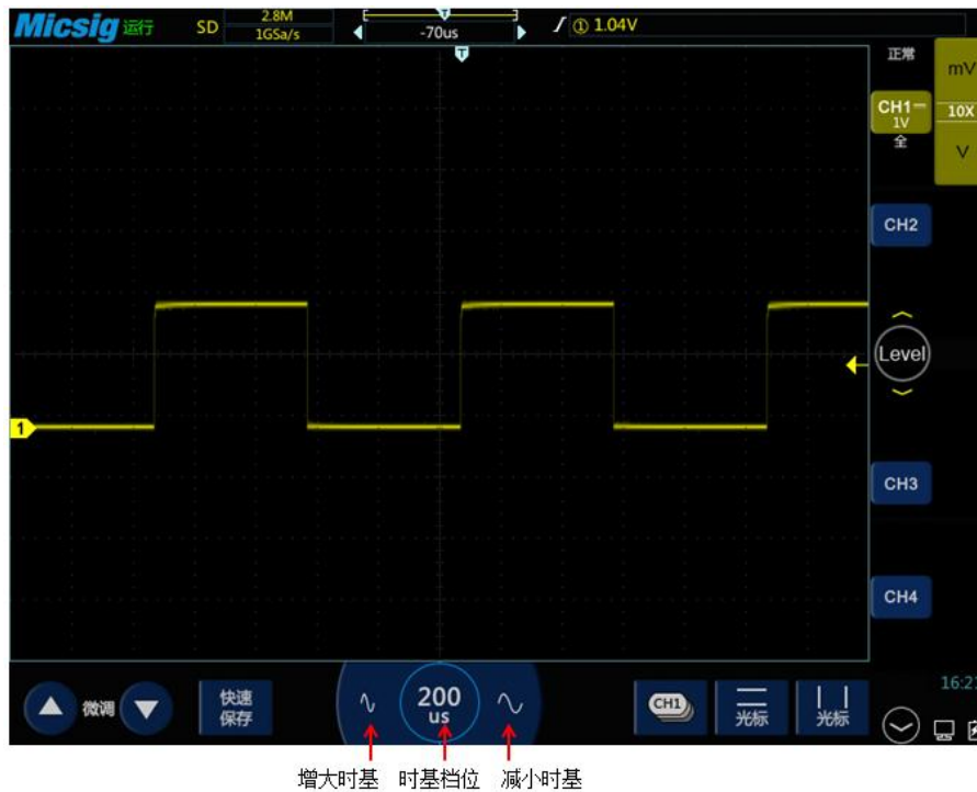
图3-3 调整水平时基
