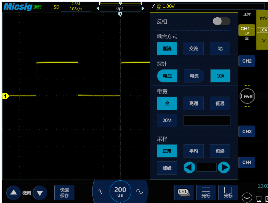
图4-8 DC耦合
