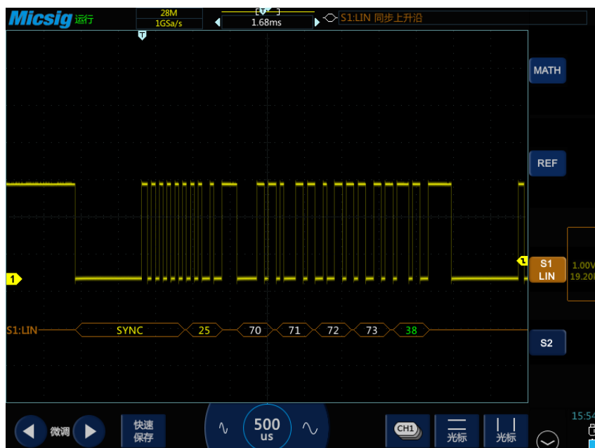
图13-8 LIN 图形界面
