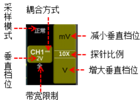
图4-3 通道显示界面
