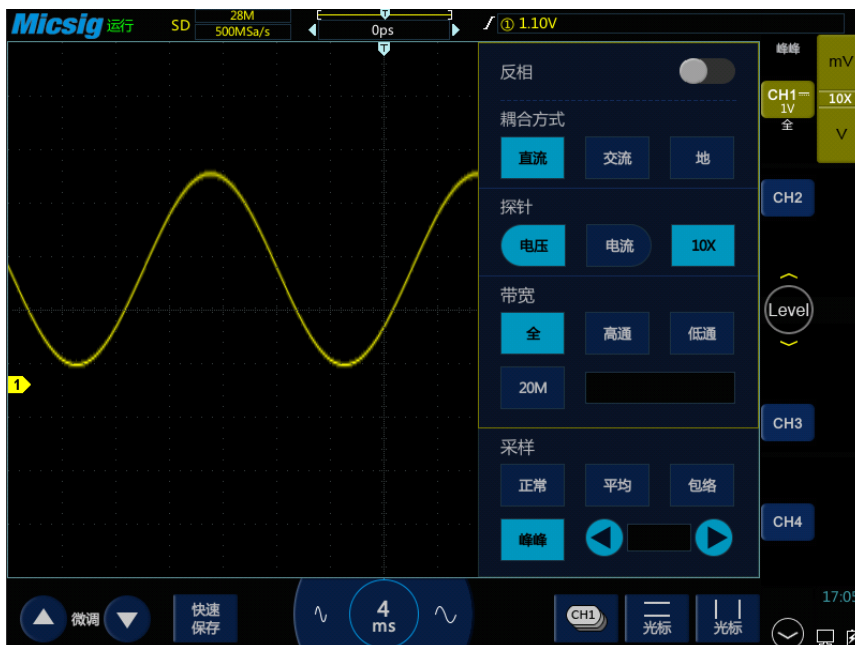
9-6 带毛刺的正弦波，峰值采样模式
