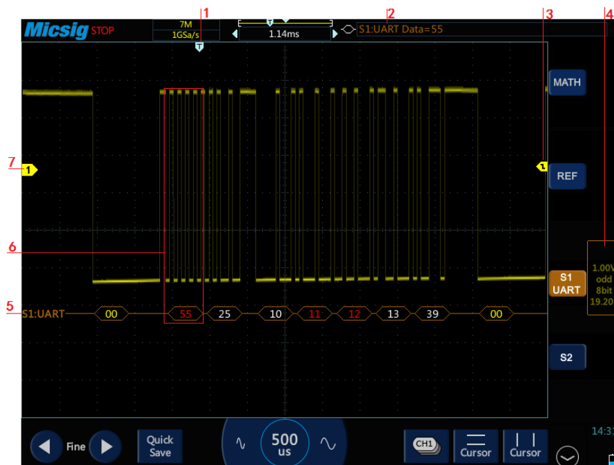
图13-5 UART 图形界面
