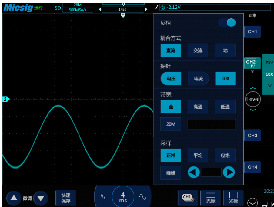
图4-13 反相后
