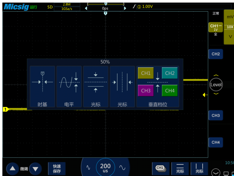
图4-6 波形垂直位置调整
