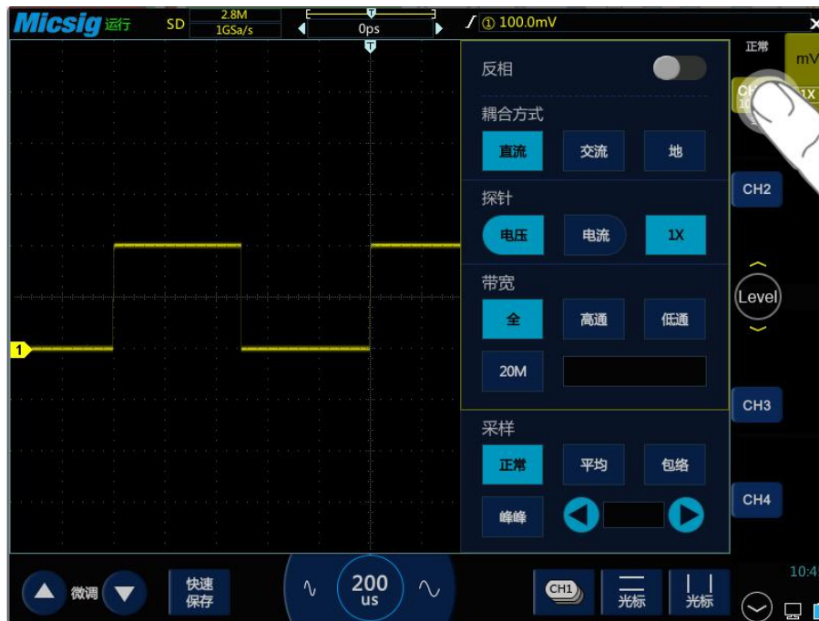
图4-7 通道切换图标及其菜单
