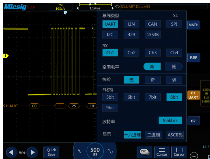
图13-2 UART 总线配置菜单
