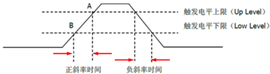
图5-25 正斜率时间/负斜率时间
