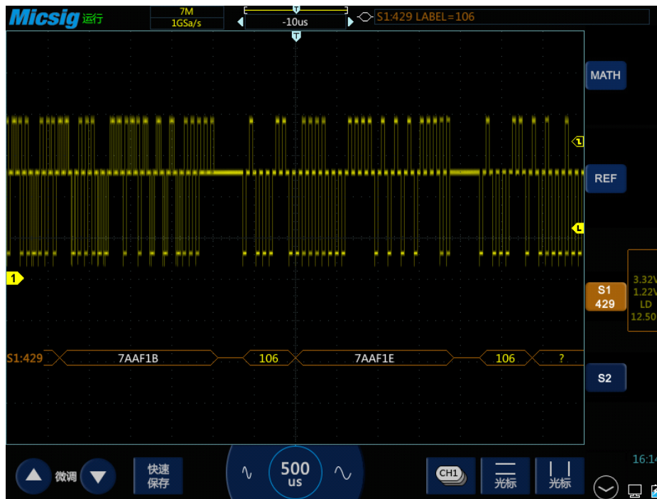
图13-20 ARINC429 图形界面
