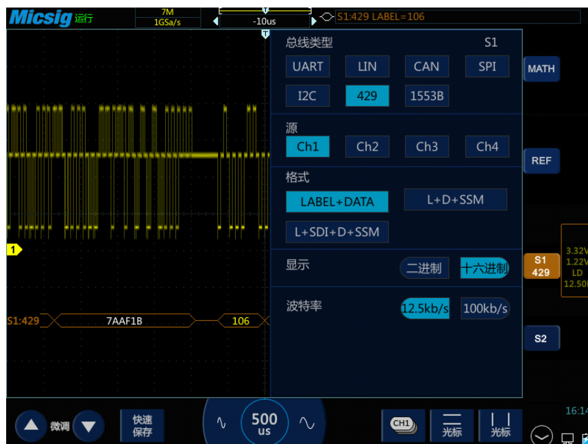
图13-18 ARINC429 总线配置菜单
