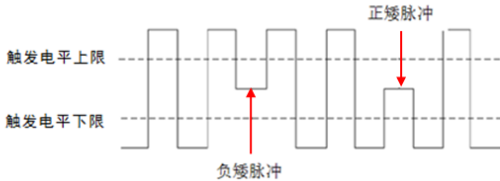
图5-23 欠幅触发
