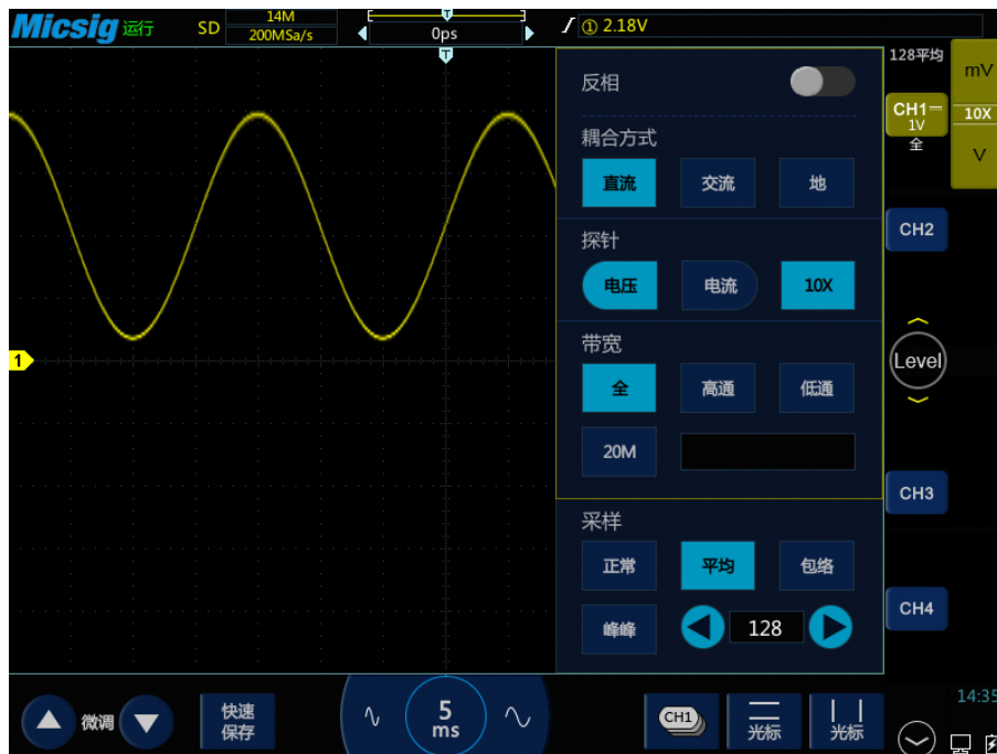
9-7 选择平均采样模式后的波形，平均数 128
