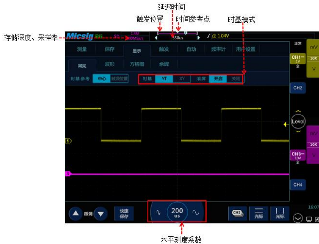
图3-1 水平系统
