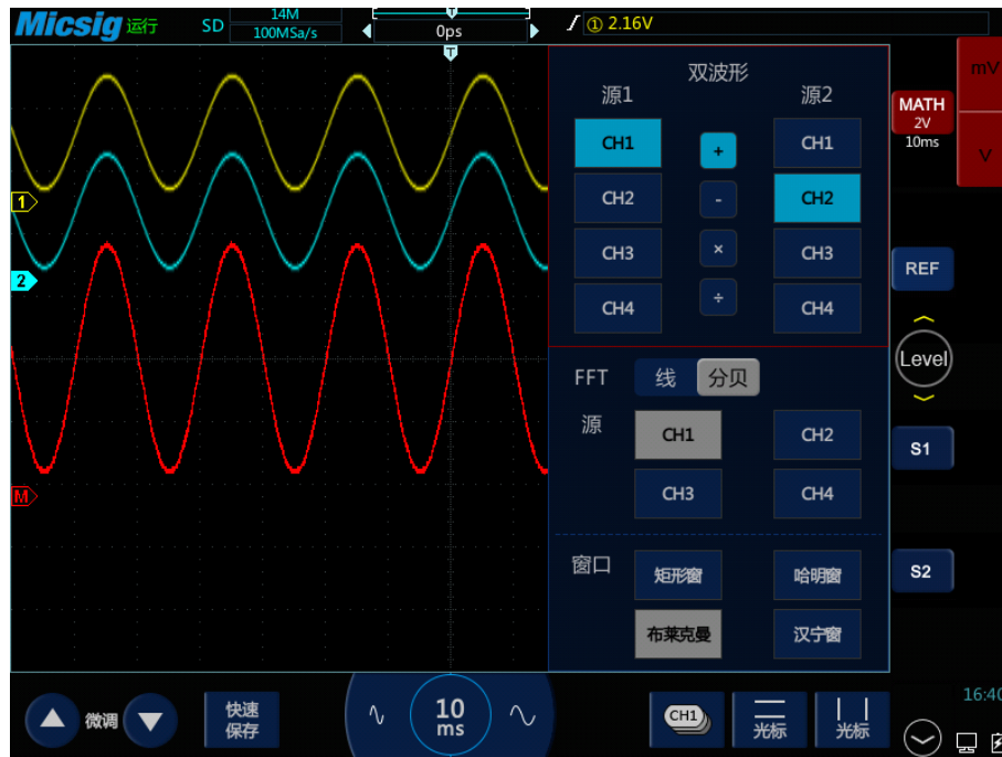
图8-1 数学通道
