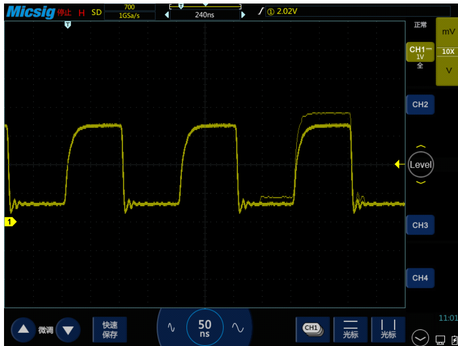
图5-3 周期信号中有异常信号
