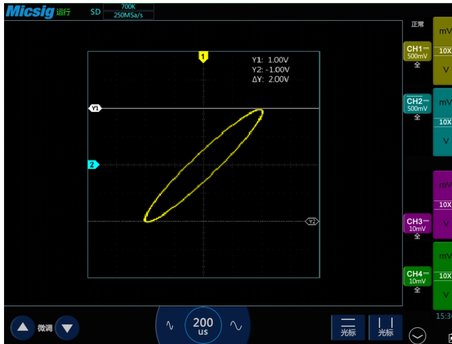
图3-9 相差测量和使用光标
