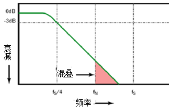
9-3 采样率和示波器带宽
