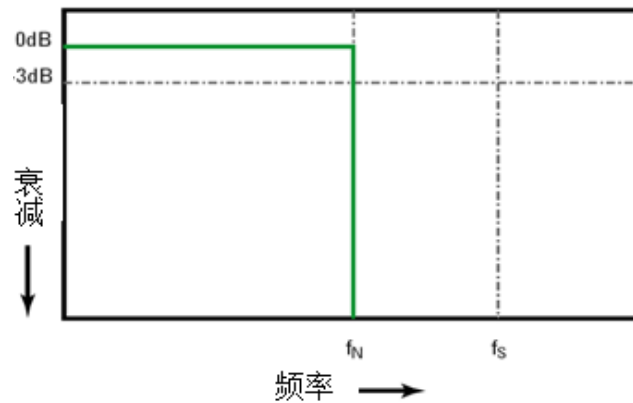
9-2 理论上的砖墙频率响应
