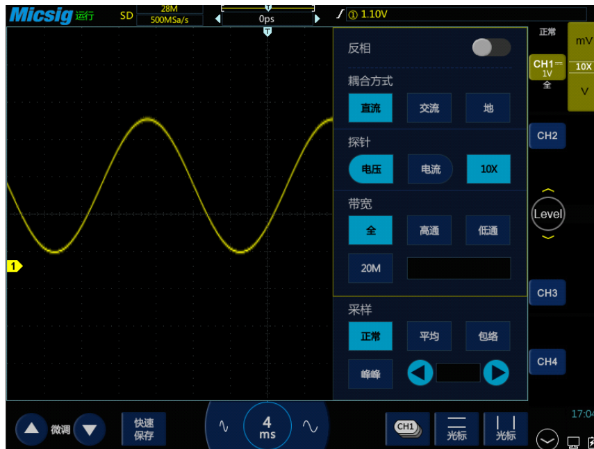
9-5 带毛刺的正弦波，正常采样模式
