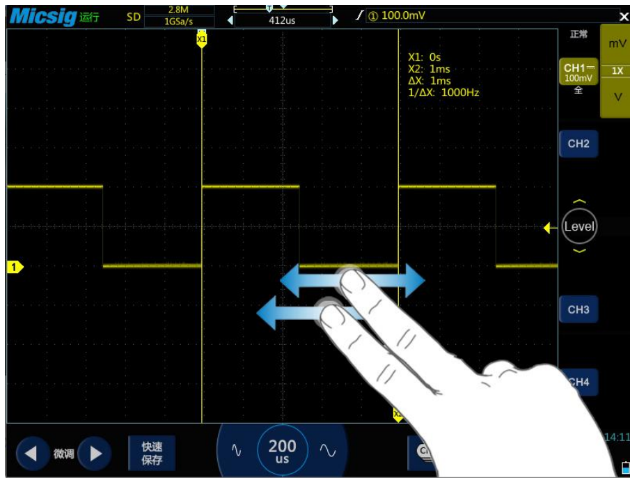
图6-11 光标测量脉冲宽度 在XY水平模式中，X光标显示CH1的值（V或A），Y光标显示CH2的值（V或A）。
