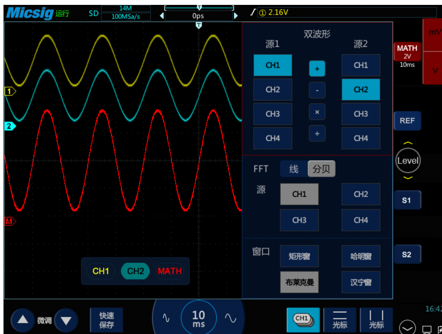
图8-2 通道 1 加通道 2 数学运算示意图
