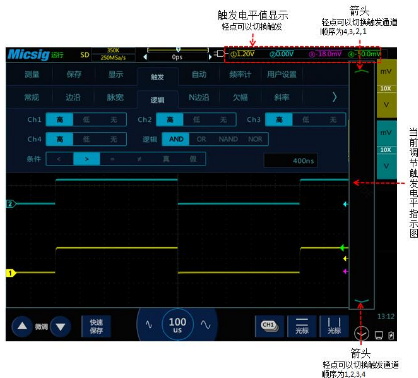
图5-21 触发电平调节
