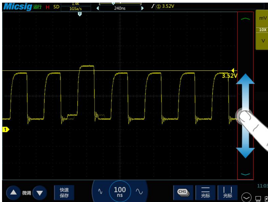
图5-4 通过设置触发电平捕获到该异常信号
