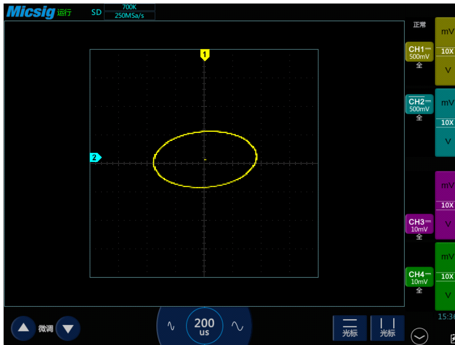
图3-7 XY 模式
