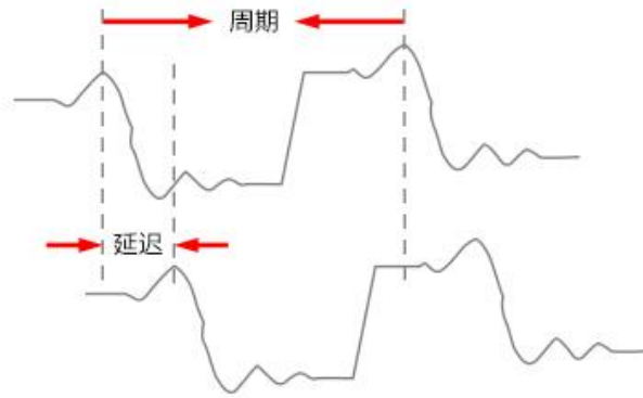
图6-6 相位测量示意图
