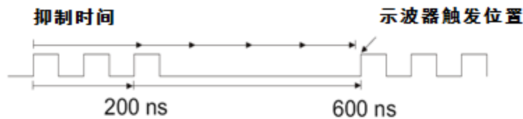
图5-9 触发抑制时间示意图说明
