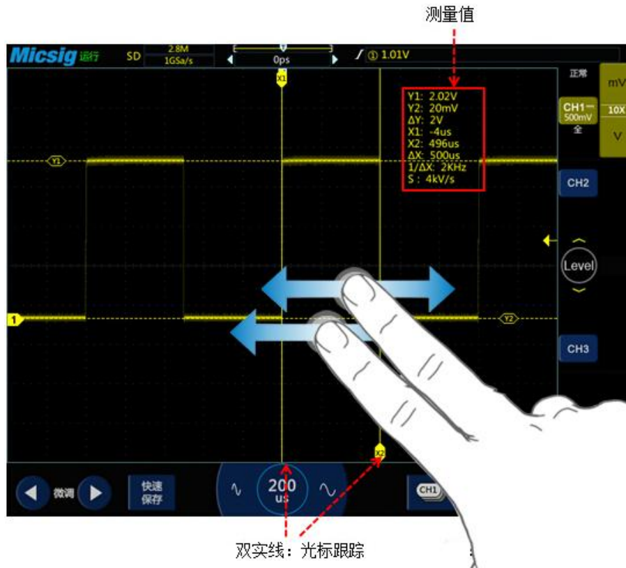
图6-9 光标测量说明
