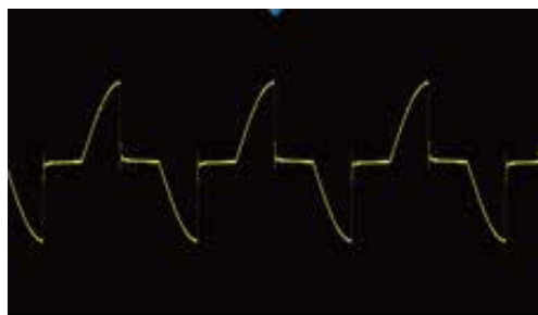
后沿TrailingEdge相位调光
