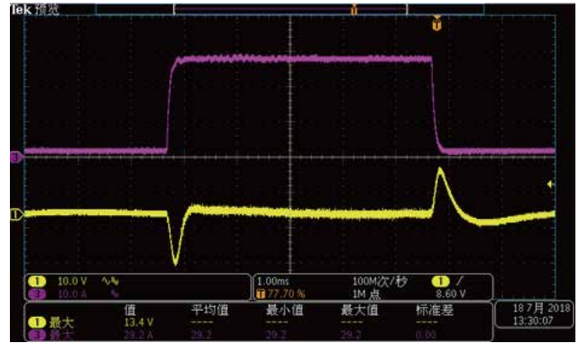
2台 IT6006B-500-30並機 設定電壓:100V, 設定電流:56A 負載電流:60A
