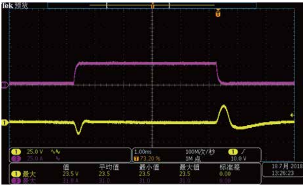
單機 IT6006B-500-30 500V 30A 6000W 設定電壓:100V 設定電流:28A 負載電流:30A
